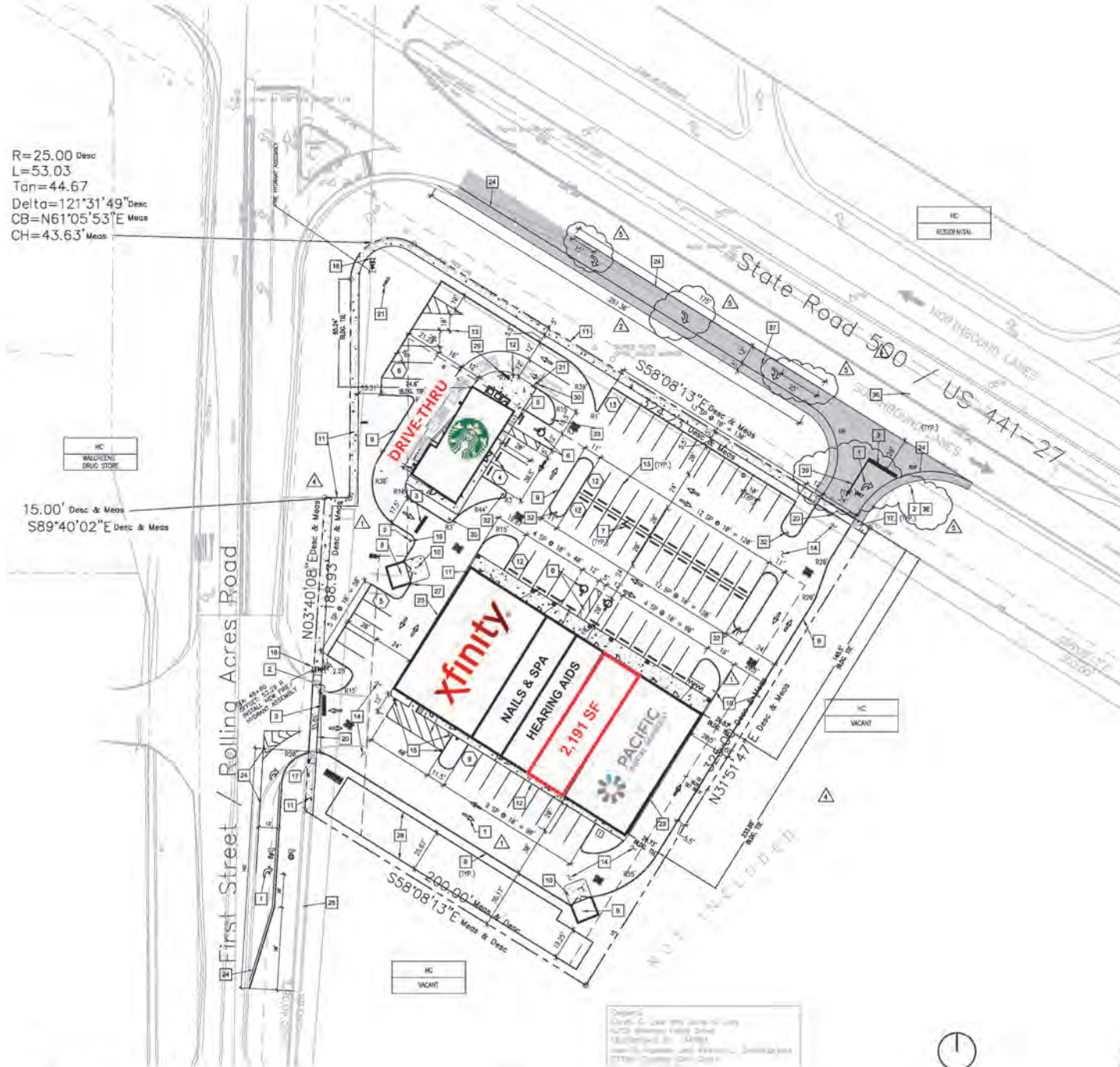
SITE DIMENSION PLAN
